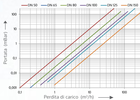
Copper-Can di serie
